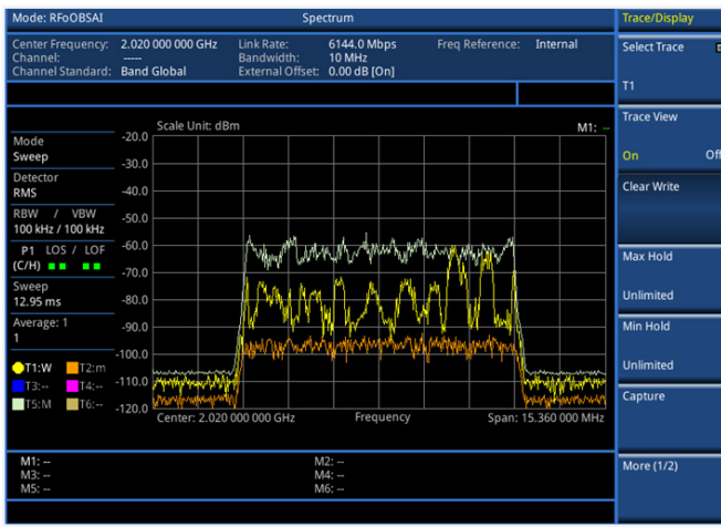
RfOBSAI – Spectrum
